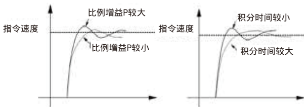
速度環 PI 參數示意圖
