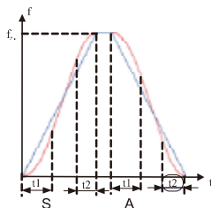
曲线加减速 示意图
