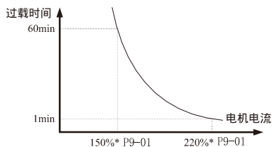
电机过载曲线
