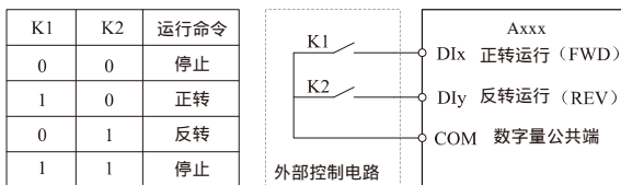
两线式模式 1
