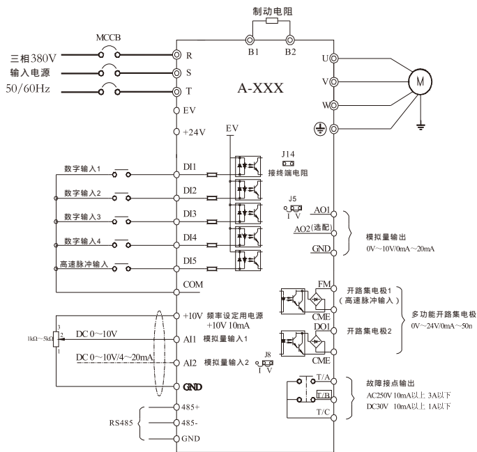
单相变频器典型接线示意
