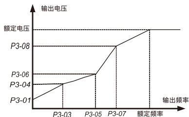
多段 V/F 示意图
