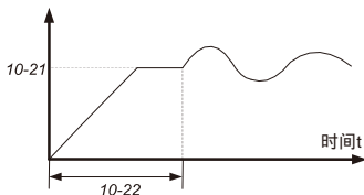
PID 预置输出示意图
