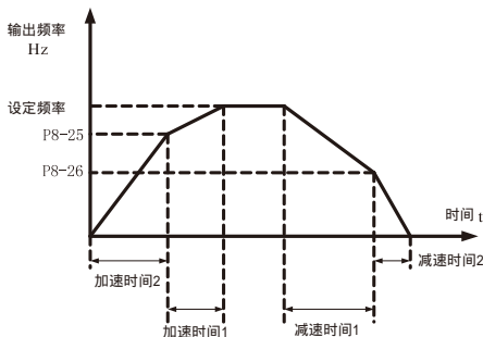
加减速时间切换示意图
