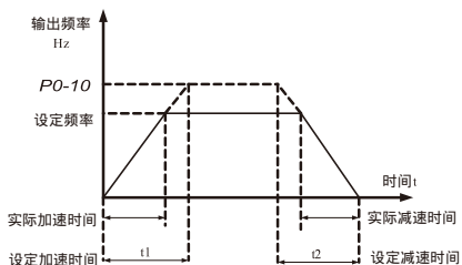
加减速时间示意图
