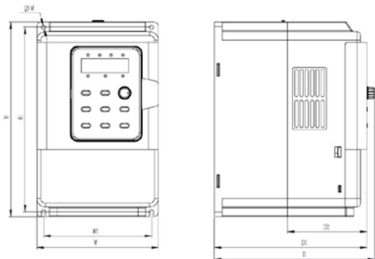
机型尺寸1
