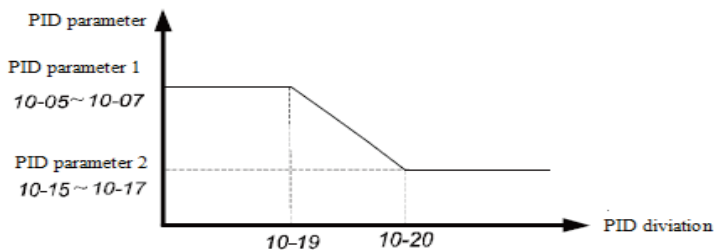
PID parameter auto switching figure
