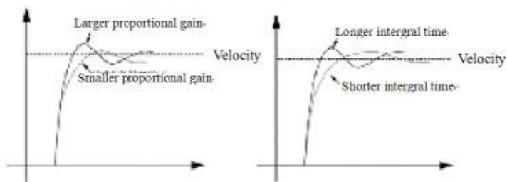
Velocity loop P1 parameter figure.
