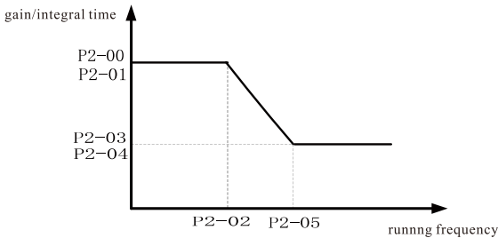
velocity loop parameter diagram
