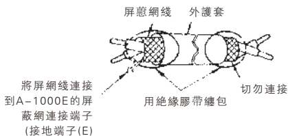
雙股屏蔽線的末端纏包
