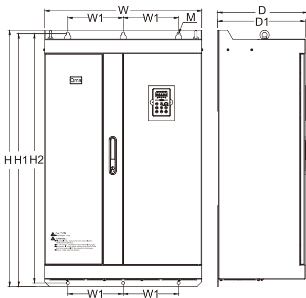
機型尺寸6
