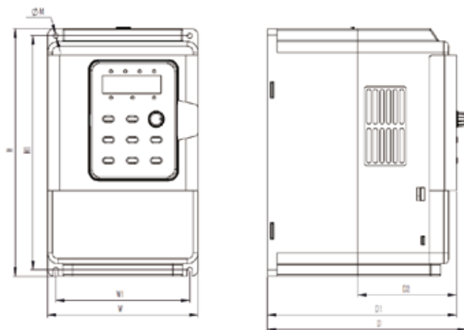
機型尺寸1
