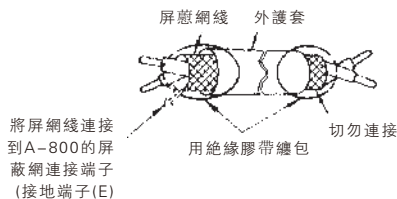
雙股屏蔽線的末端纏包
