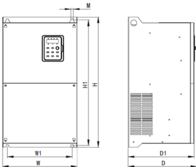
機型尺寸4
